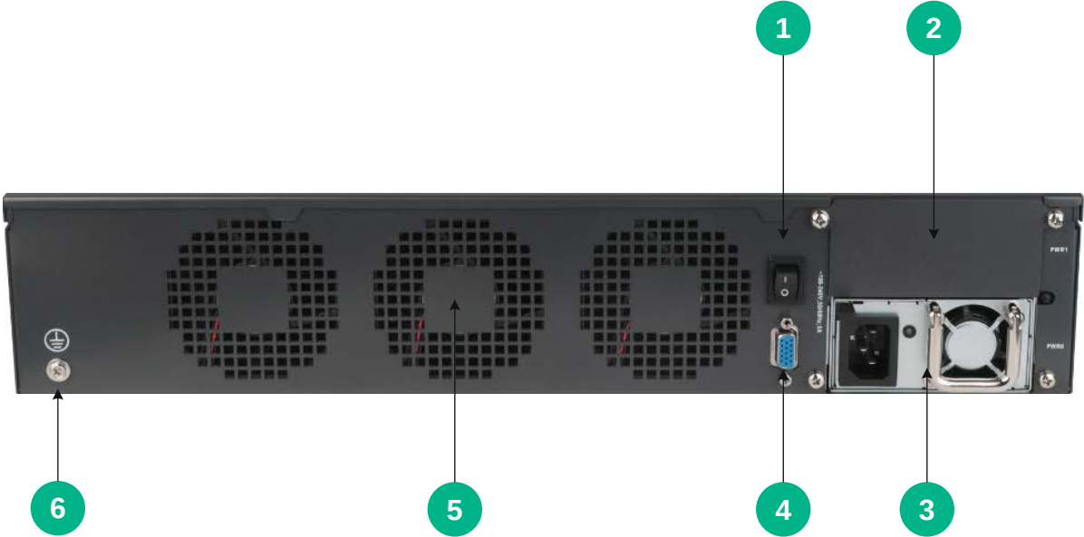
图A-4 UNIS XScan-G20 设备后视图
