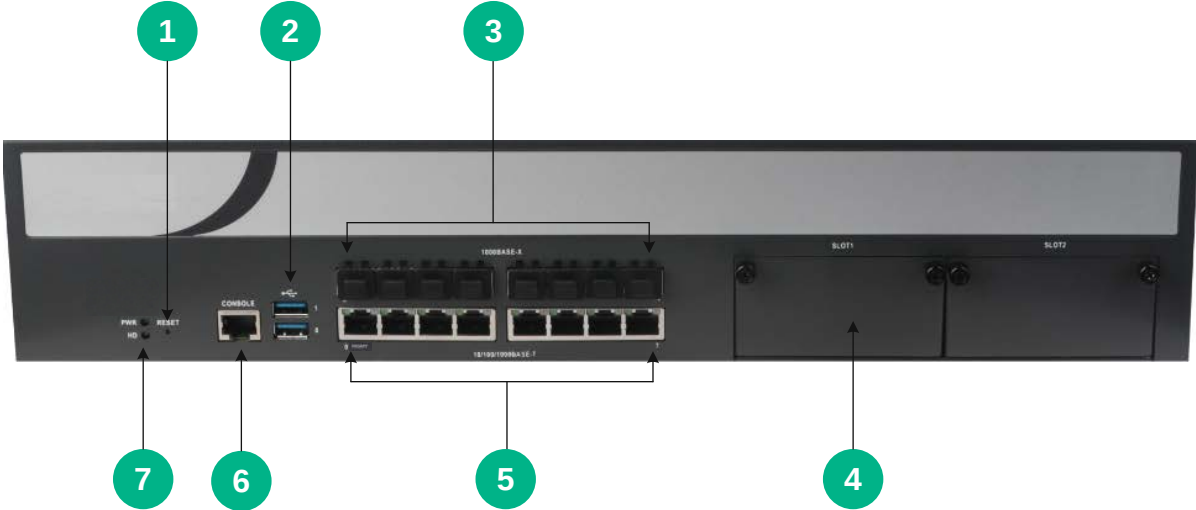
图A-3 UNIS XScan-G20 设备前视图
